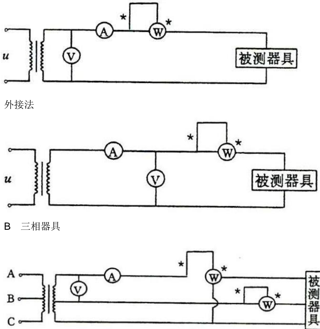
图 4-1 输入功率测量（稳态）
