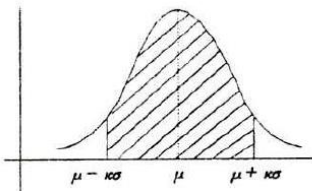
图 4-3 正态分布
