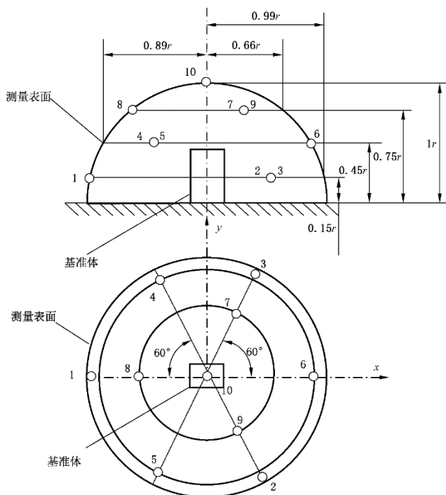
图 A6-1 半球面测量表面布点图
