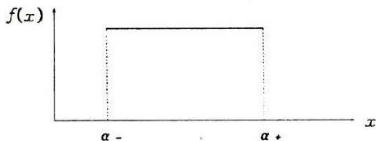
图 4-4 均匀分布
